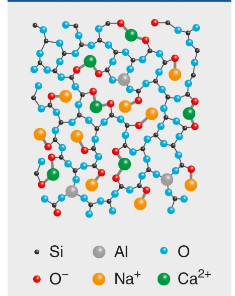
NORMALGLAS
