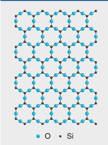
QUARZKRISTALL ( \text{SiO}_2 )
