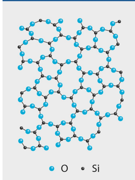
QUARZGLAS ( \text{SiO}_2 )
